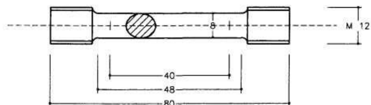
Образец для испытания на растяжение
