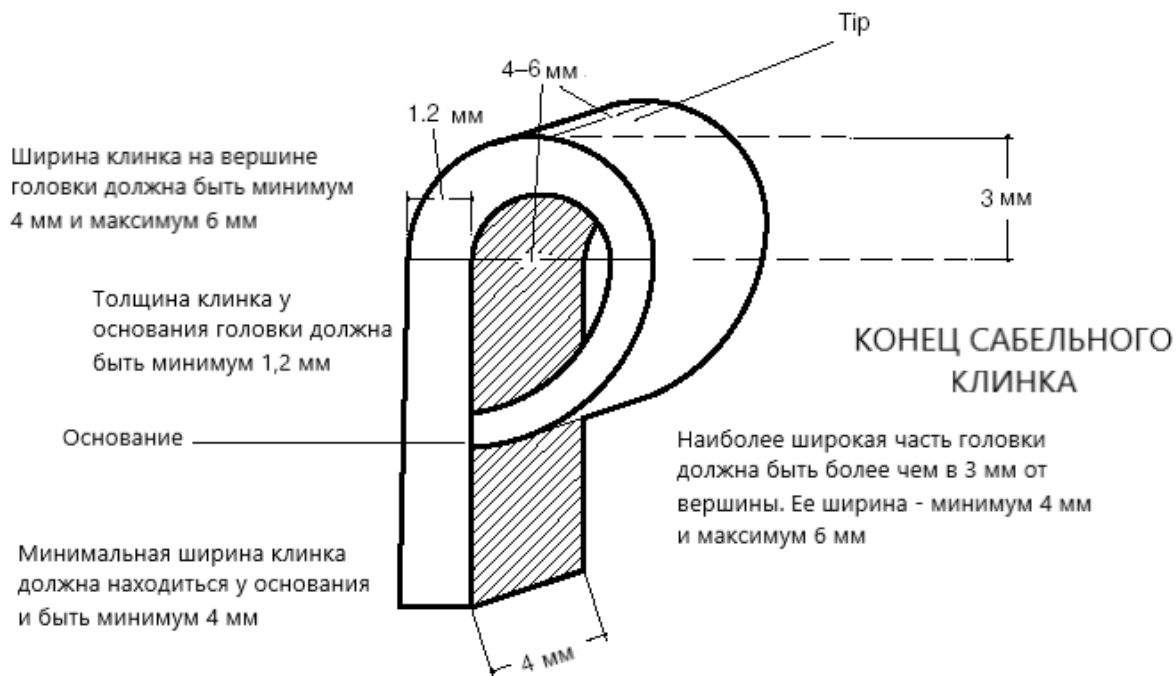
Рис. 12. Размеры и гибкость сабли.
