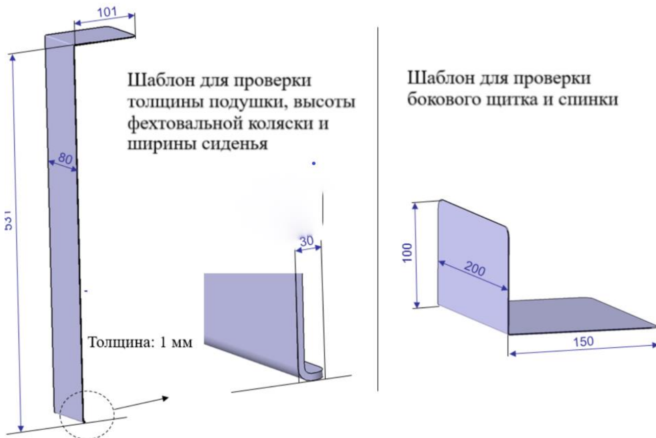
Рис. 13.2. Шаблоны для тестирования фехтовальной коляски
