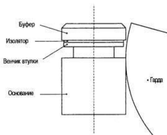
Рис. 11. Шпага: детали кнопки наконечника
