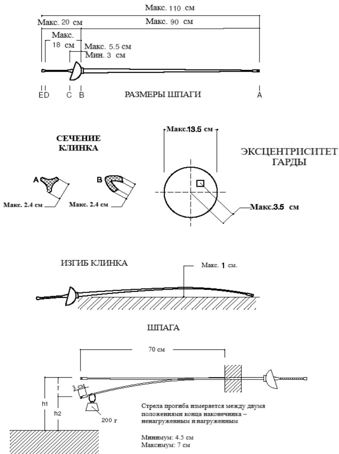
Рис. 9. Размеры и гибкость шпаги.
